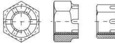
DIN 937 CASTLE NUTS
