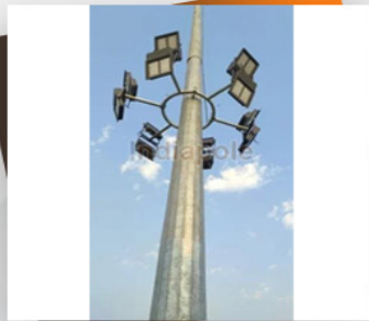
12 Meter High Mast Pole
