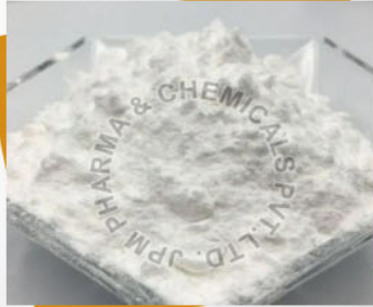
Atenolol
