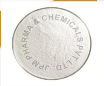
Bromhexine HCL
