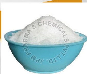
Cyclohexanol
