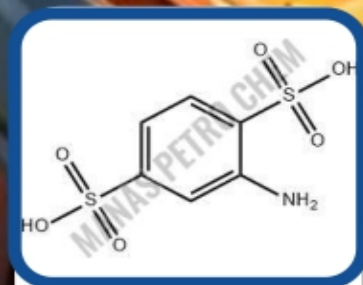
1,3 Benzenedisulfonic Acid, 4 - Amino 137-
