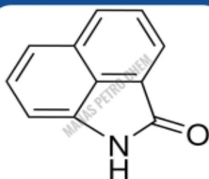
Benz (cd) Indol- 2 (1H)-One
