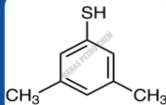
3,5-Dimethylbenzenethiol
