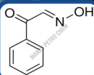
2-Isonitrosoacetophenone
