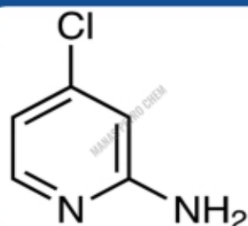
2-Amino-4-chloropyridine
