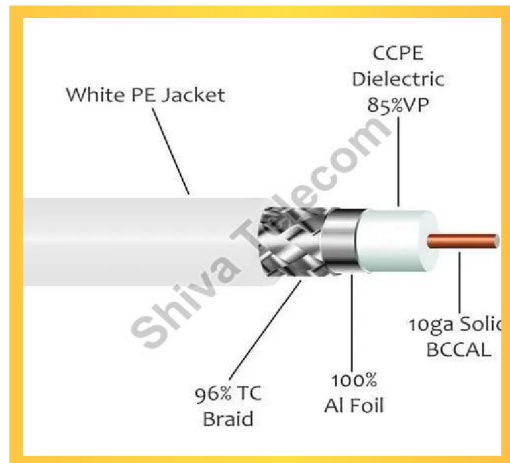
RG 6 Cable
