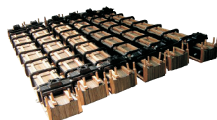
Furnace Yoks
