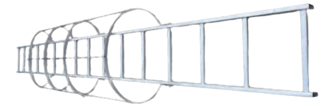
Long Ladder for K Mast Section K 标准节梯子
