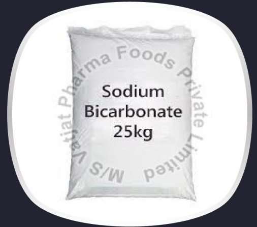
Sodium Bicarbonate
