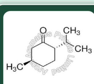
Menthone (70:30)
