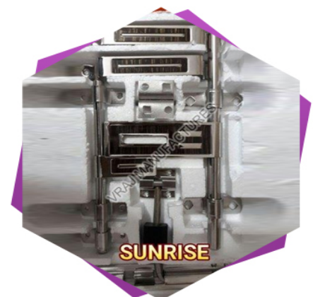
Mica Door Kit
